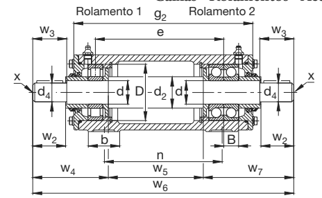
VRE3... C
