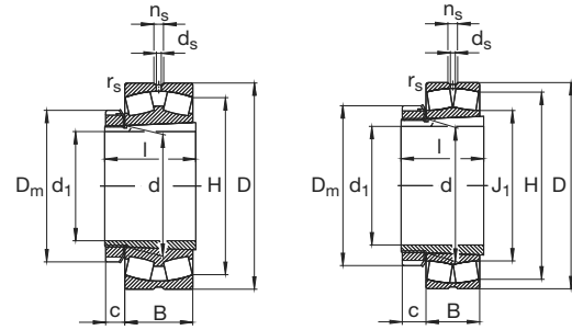
Construção E
