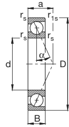
B719E, B70E, B72E Ângulo de contato \alpha = 25^\circ
