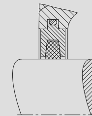
Vedação de feltro
