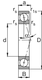
B719C, B70C, B72C Ângulo de contato \alpha = 15^\circ
