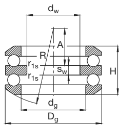
542, 543 Anéis de caixa esféricos
