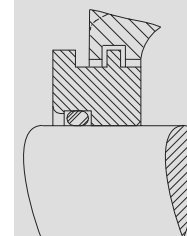
Vedação de labirinto radial
