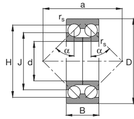
33DA anel interno bipartido Ângulo de contato \alpha = 45^\circ
