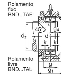
Execução A
