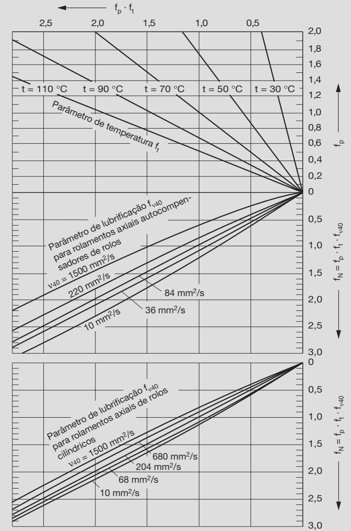
▼ Diagrama 6: parâmetro de temperatura f_t para rolamentos axiais de rolos (em cima), parâmetro de lubrificação f_{v40} e relação de rotação f_N (em baixo) para rolamentos axiais autocompensadores de rolos, (meio), e para rolamentos axiais de rolos cilíndricos (em baixo), para a determinação da rotação em serviço termicamente permitida
