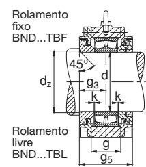
Execução B
