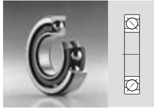
Rolamento de contato angular de esferas de uma carreira
