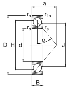
B Ângulo de contato \alpha = 40^\circ
