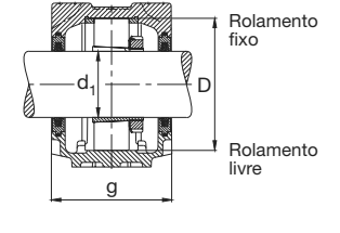
Vedação de feltro FSV
