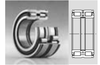
Rolamento de rolos cilíndricos de duas carreiras, sem gaiola
