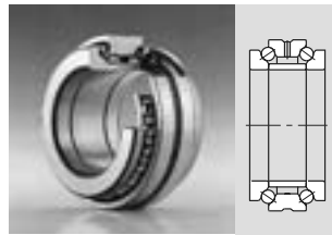
Rolamento axial de contato angular de esferas de escora dupla
