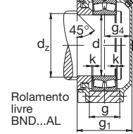
Execução A
