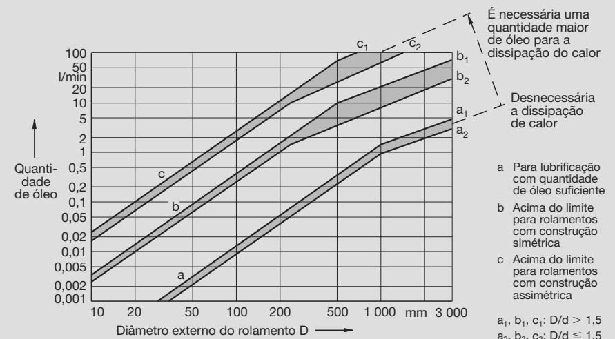
▼ Quantidades de óleo na lubrificação por recirculação
