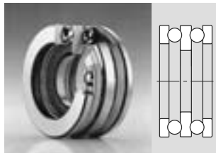
Rolamento axial de esferas de escora dupla
