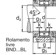
Execução B
