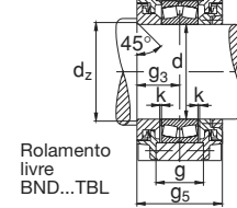
Execução B
