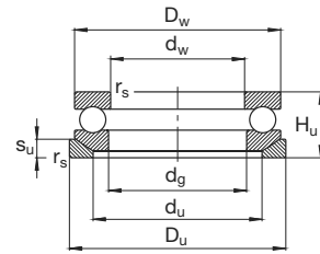
532, 533 Anel de caixa esférico e contraplaca U2, U3
