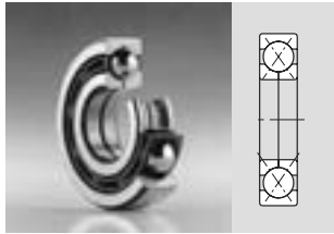
Rolamento de quatro pistas
