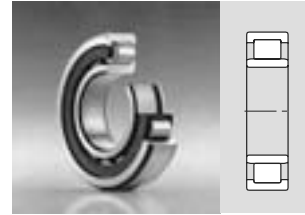
Rolamento de rolos cilíndricos de uma carreira
