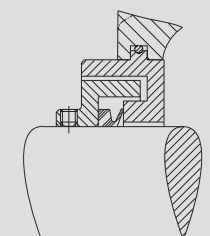
Vedações combinadas de contato (Taconite)
