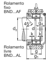
Execução A
