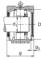
Vedação de dois lábios DH Tampa DKV
