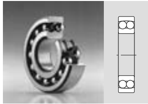
Rolamento autocompensador de esferas
