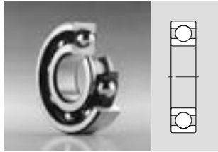
Rolamento fixo de esferas de uma carreira
