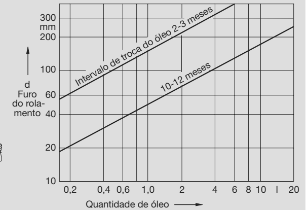
▼ Quantidade de óleo e intervalos para a troca, dependendo do furo do rolamento
