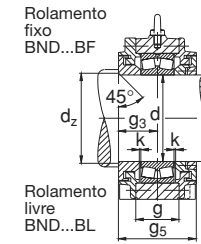
Execução B
