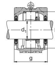
Vedação de feltro FSV
