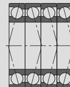
QBT Combinação da disposição em O e em Tandem
