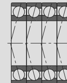
QTT Disposição em Tandem
