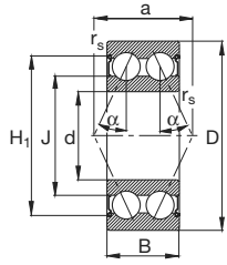
32B, 33B Ângulo de contato \alpha = 25^\circ
