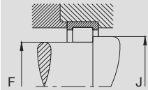
▼ Medidas de montagem para a execução RNU sem o anel interno
