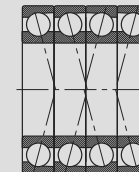
QFC Disposição em X
