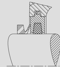
Vedação de feltro + anel V
