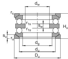
542, 543 Anéis de caixa esféricos e contraplacas U2, U3
