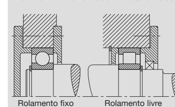
Rolamento fixo Rolamento livre
