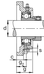
F162
