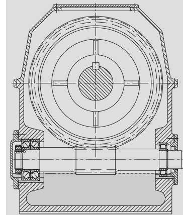
▼ Nível do óleo na lubrificação por imersão
