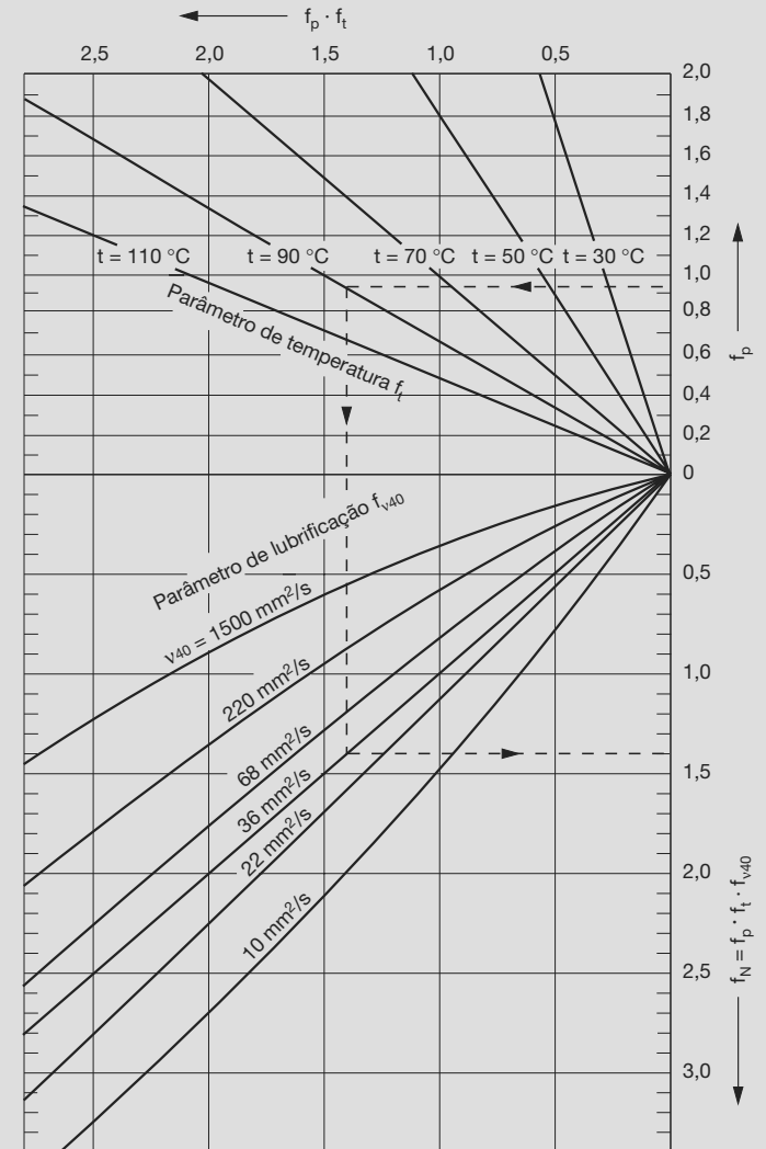
▼ Diagrama 2: parâmetro de temperatura f_t (em cima), parâmetro de lubrificação f_{v40} e relação de rotação f_N (em baixo) para rolamentos radiais de esferas, para a determinação da rotação em serviço termicamente permitida
