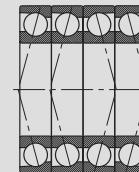
QBC Disposição em O
