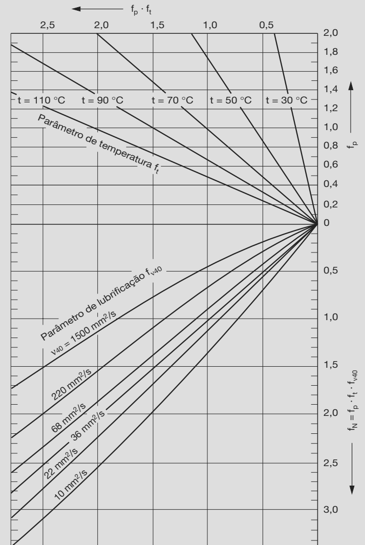
▼ Diagrama 4: parâmetro de temperatura f_t (em cima), parâmetro de lubrificação f_{v40} e relação de rotação f_N (em baixo) para rolamentos radiais de rolos para a determinação da rotação em serviço termicamente permitida
