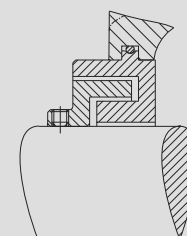
Vedação de labirinto axial
