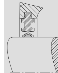
Vedação de dois lábios
