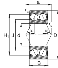
32B.2RSR, 33B.2RSR
