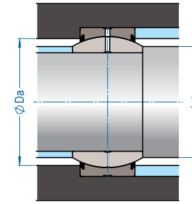
GE(00)FO 2RS dimensões de montagem
